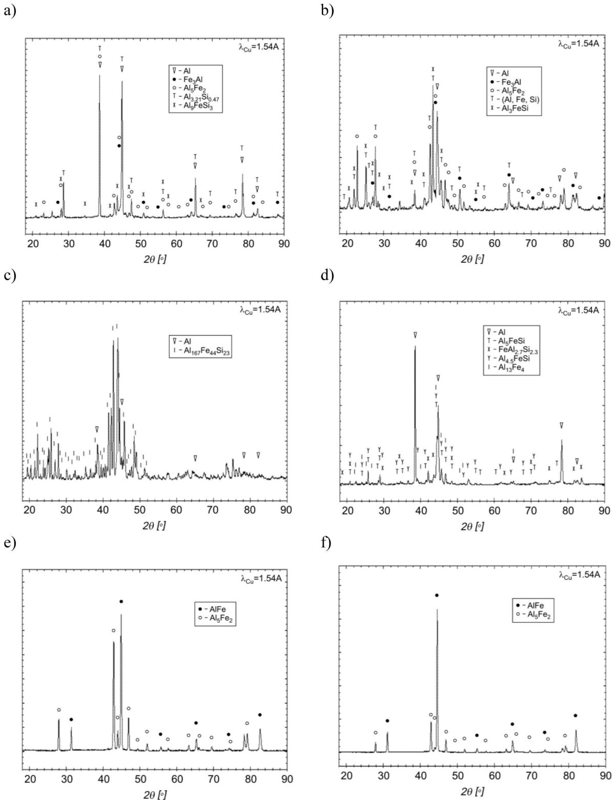
Fig. 9. Results of the X-ray phase analysis a) 500°C - 1440min., b) 600°C - 30min., c) 700°C - 5min., d) 900°C - 1min., e) 950°C - 5min., f) 1000°C - 5min
